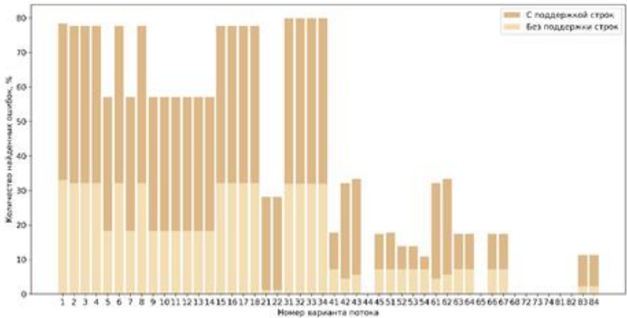
Рис. 2. Срабатывания анализатора на различных вариантах потока Fig. 2. Reported warnings by flow variants
