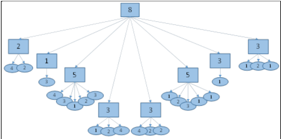
Рис. 4. Структура декомпозиции модели OLAP-системы.
