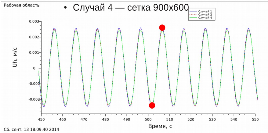
Рисунок 16. Сравнение сеточного разрешения и схема выбора точек для кросс-тестирования МКО и МСЭ
