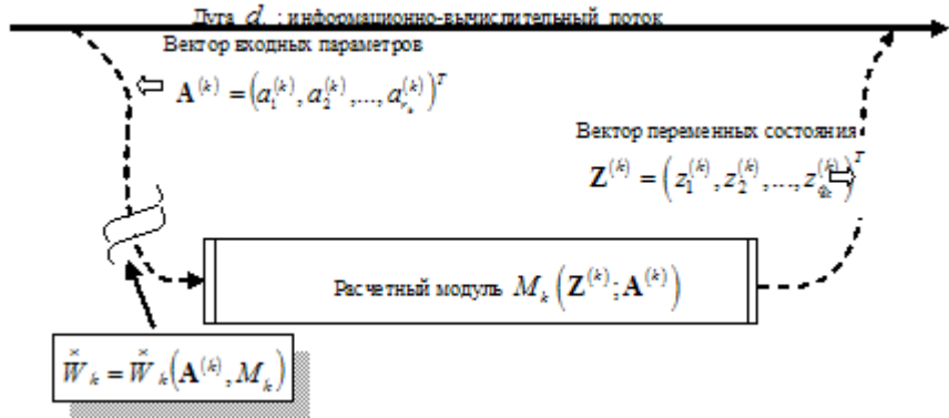
Рисунок 1. Вычислительная нагрузка дуги орграфа
