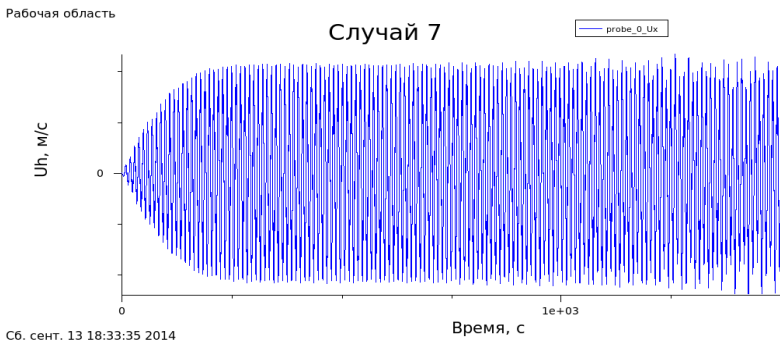
Рисунок 11. Динамика горизонтальной составляющей скорости в точке (28.2, 20) для случая 7 (без постепенного вывода скорости движения подвижной стенки)
