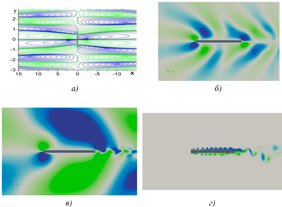
Рис.1. Структура стратифицированного течения( N=1.2c^{-1} ) около неподвижной (а – течение, индуцированное диффузией) и равномерно движущейся(б – Re=10^3 в Re=5 \cdot 10^3 , г – Re=8 \cdot 10^4 ) горизонтальных пластин( L = 10 см, h = 0.5 см).
