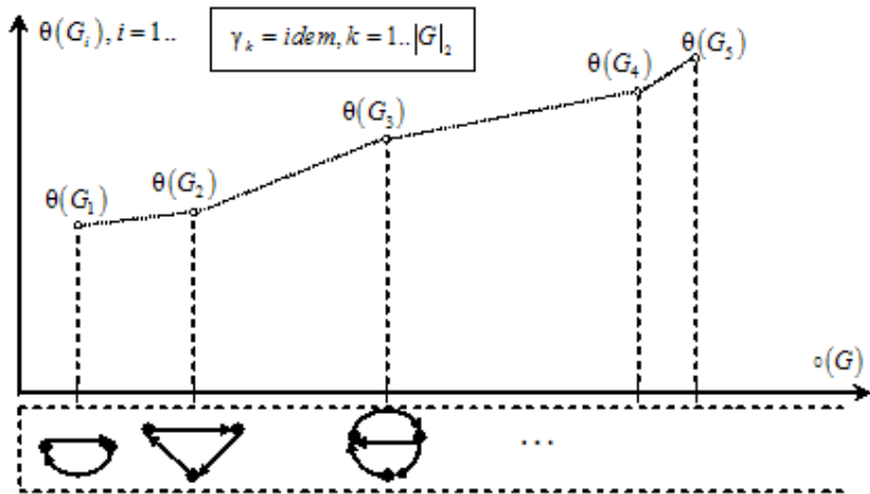
Рисунок 2. Иллюстрация к гипотезе о росте оценок сложности орграфов при их лексикографическом перечислении в условиях постоянства параметрических
