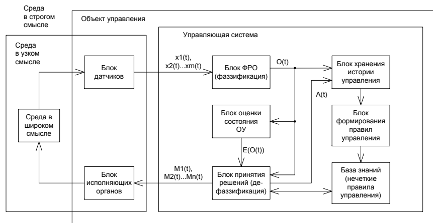
Рис. 2. Общая структура системы ААУ с использованием нечеткой логики.
