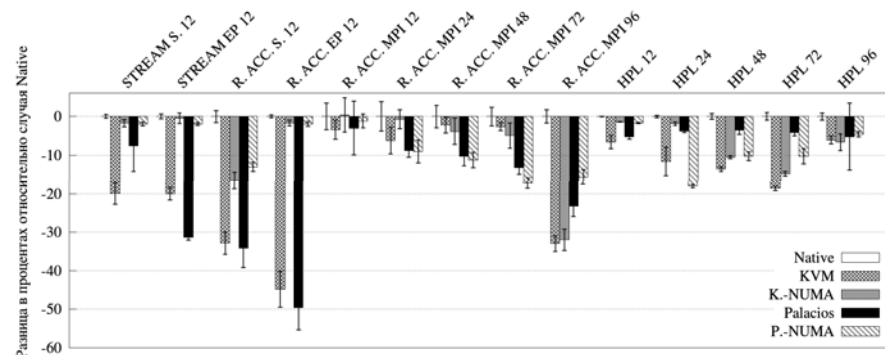
Рис. 5. Результаты KVM/QEMU и Palacios для тестов пакета HPCC.
