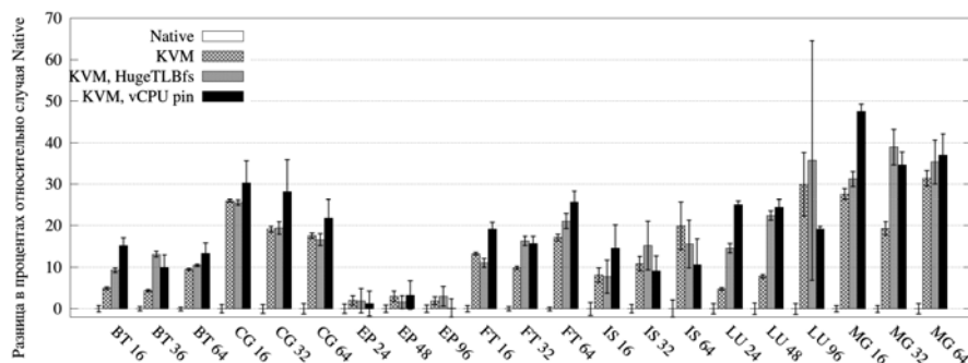
Рис. 1. Первичные результаты KVM/QEMU на тестах пакета NPВ.
