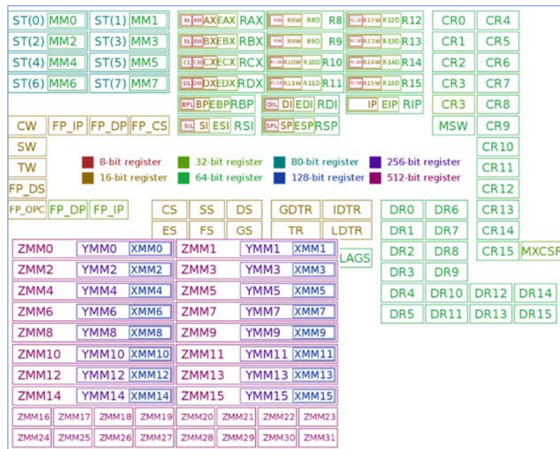
Рис. 1. Регистры x64 Fig. 1. x64 registers
